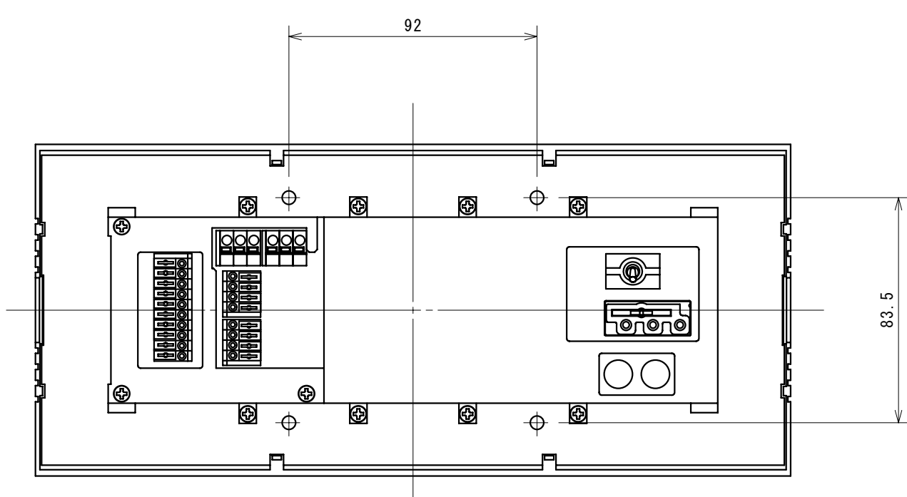
背面図
